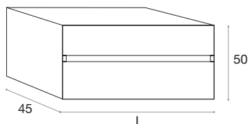
Cassetiera su ruote - alt. 50cm, prof. 45cm Unit on wheels - height 50cm, depth 45 cm
