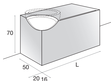
Scarico a parete - versione a parete Siphon on the wall - on the wall version
