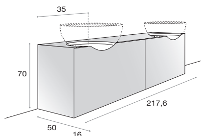
Scarico a parete - versione a parete Siphon on the wall - on the wall version
