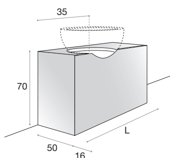
Scarico a parete - versione a parete Siphon on the wall - on the wall version
