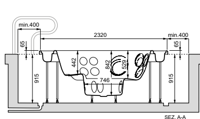
SEZ. A-A
