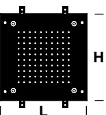
Piastra soffione incasso 430X430 con nebulizzatori 430x430 built-in ceiling plate with nebulizers
