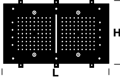
Piastra soffione incasso 700X400 con cascata, cromoterapia e nebulizzatori | 700x400 built-in ceiling plate with waterfall, chrome therapy and nebulizers
