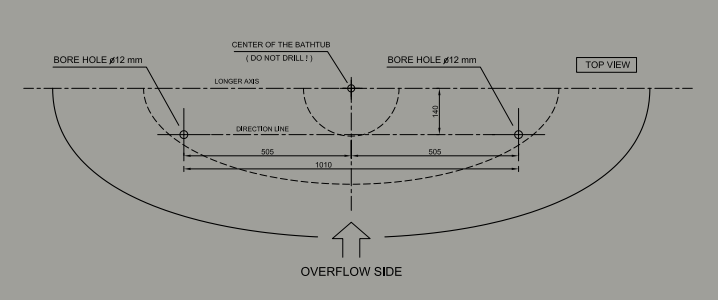
НАПОЛЬНОЕ КРЕПЛЕНИЕ И УСТАНОВКА Напольное крепление – уникальная концепция напольного крепления отдельностоящих ванн! Набор состоит из 2 шурупов, 2 болтов, 2 предварительно собранных отверстий, что гарантирует устойчивое положение ванны на полу. Каждая ванна поставляется с подробным шаблоном для сверления пола и наглядной схемой инструкцией по монтажу.
