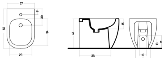
Bidet a terra in ceramica bianca Free standing bidet in white ceramic / WC aus weißer Keramik Bidet au sol en céramique blanche / Биде напольное из белой керамики
