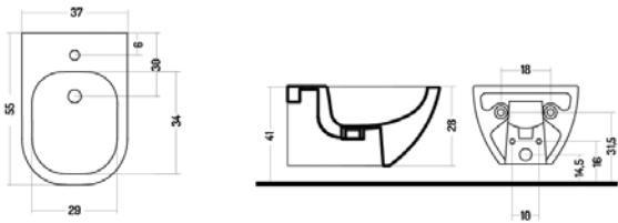
Bidet sospeso in ceramica bianca Wall-hung bidet in white ceramic / Hängendes Bidet aus weißer Keramik Bidet suspendu en céramique blanche / Биде подвесное из белой керамики
