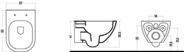
WC sospeso in ceramica bianca, completo di sedile bianco a chiusura rallentata Wall-hung WC in white ceramic, complete with soft close toilet seat Hängendes WC aus weißer Keramik mit weißem Sitz und gedämpfter Schliessung WC suspendu en céramique blanche, avec siège blanc à fermeture ralentie унитаз подвесной из белой керамики в комплекте с белым сиденьем, оснащенный механизмом плавного опускания крышки
