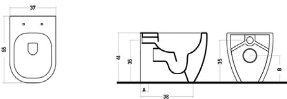
WC a terra in ceramica bianca, completo di sedile bianco a chiusura rallentata Free standing WC in white ceramic, complete with soft close toilet seat WC aus weißer Keramik mit weißem Sitz und gedämpfter Schliessung WC au sol en céramique blanche, avec siège blanc à fermeture ralentie унитаз напольный из белой керамики в комплекте с белым сиденьем, оснащенный механизмом плавного опускания крышки
