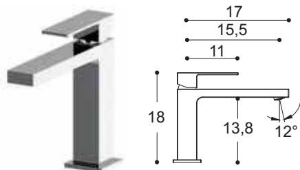
one-hole tap, without drain pipe mitigeur vasque monotrou, sans bonde
