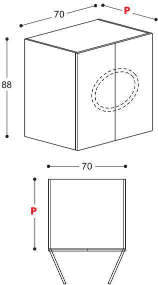
Washing machine cabinet with two hinged doors Élément bas pour machine à laver avec deux portes battantes
