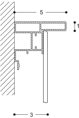
mirror with top and bottom led, with frame in lacquered aluminium H. 70 cm miroir avec led supérieure et inférieure, avec cadre en aluminium laqué H. 70 cm
