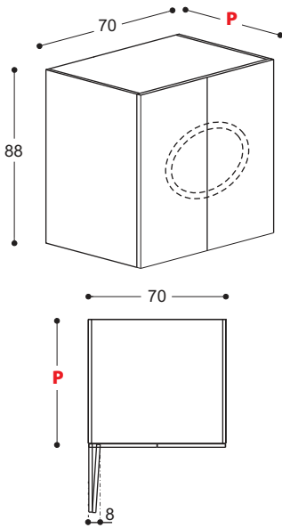
Washing machine cabinet with two folding doors Élément bas pour machine à laver avec deux portes pliantes
