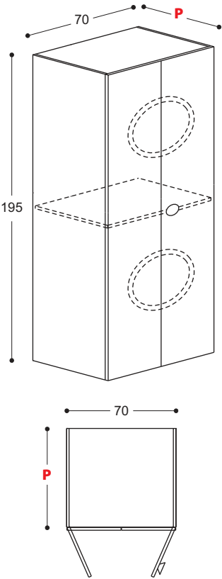
Washing machine column with two hinged doors Colonne pour machine à laver avec deux portes battantes
