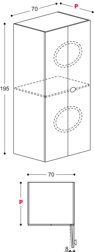
Washing machine column with two folding doors Colonne pour machine à laver avec deux portes pliantes
