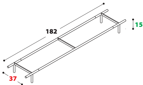
metal base base de métal
