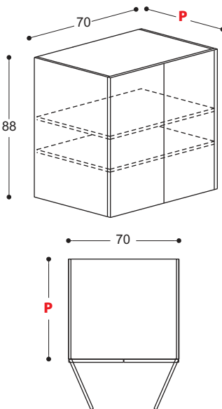
Base cabinet with 2 shelves and two hinged doors Élément bas avec 2 tablettes et deux portes battantes
