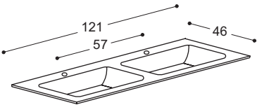
plan vasque moulée double en céramique 2 vasques 47x28xh12 integrated double Ceramic w-b 2 wash-basins 47x28xh12
