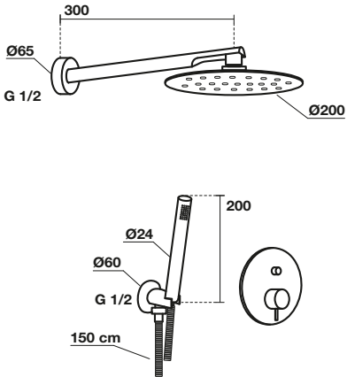
9231 Kit doccia miscelatore con deviatore, doccetta, braccio e soffione Ø20 Mixer shower faucet kit w/diverter, handshower, rod and showerhead Ø20
