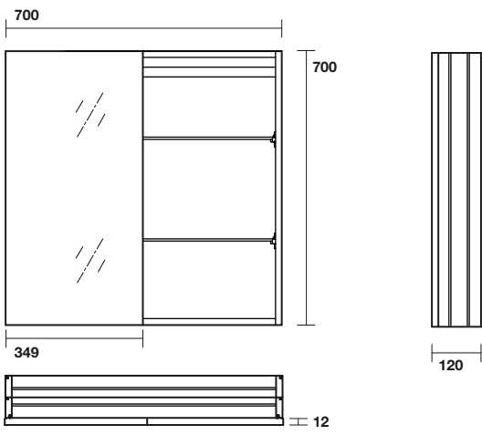
9215 Specchio contenitore in alluminio 70x70 con due ante e due ripiani interni Alluminium mirror cabinet 70x70 two door and two inner shelves
