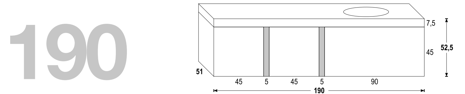
PORTALAVABO SOSPESO SENZA TOP - L. 190 P.51 H. 52,5 WALL-MOUNTED WASHBASIN CABINET WITHOUT TOP - W.190 D.51 H.52,5
