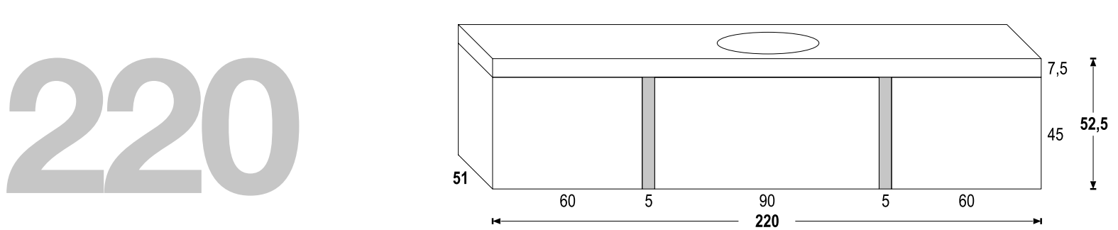
PORTALAVABO SOSPESO SENZA TOP - L. 220 P.51 H. 52,5 WALL-MOUNTED WASHBASIN CABINET WITHOUT TOP - W.220 D.51 H.52,5
