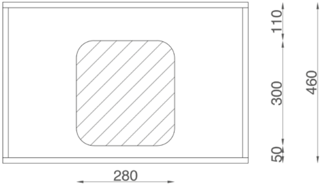
LAVABI MUTEVOLE - VISTA IN PIANTA MUTEVOLE BASINS - PLAN VIEW
