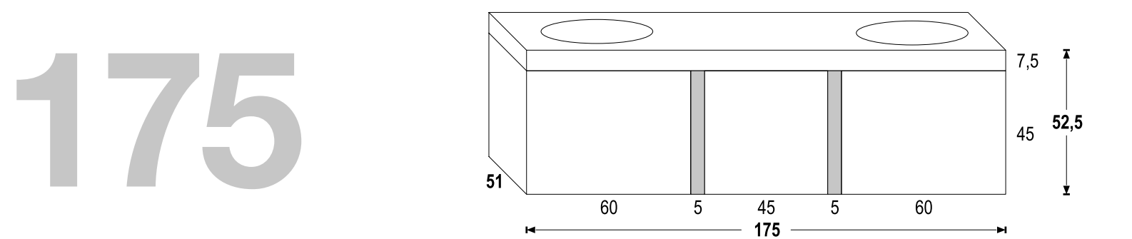
PORTALAVABO SOSPESO SENZA TOP - L. 175 P.51 H. 52,5 WALL-MOUNTED WASHBASIN CABINET WITHOUT TOP - W.175 D.51 H.52,5
