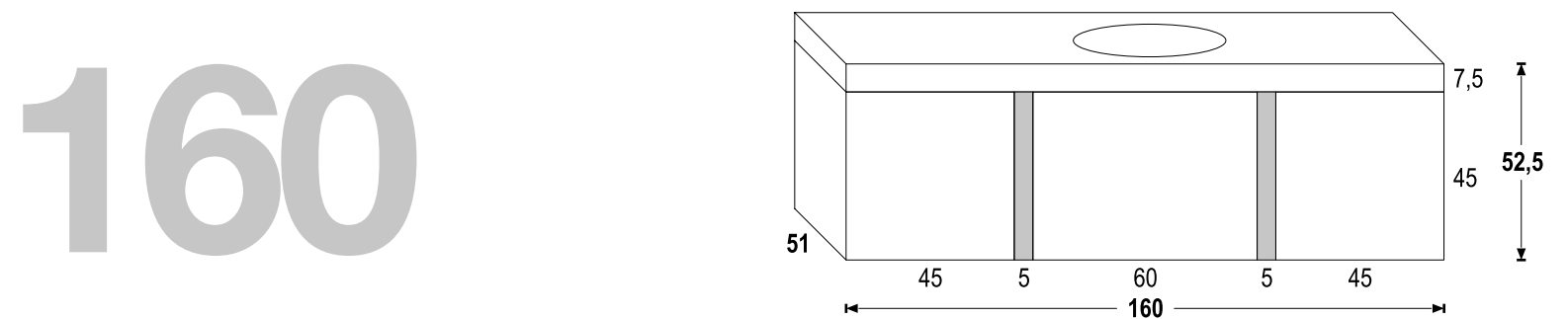
PORTALAVABO SOSPESO SENZA TOP - L. 160 P.51 H. 52,5 WALL-MOUNTED WASHBASIN CABINET WITHOUT TOP - W.160 D.51 H.52,5
