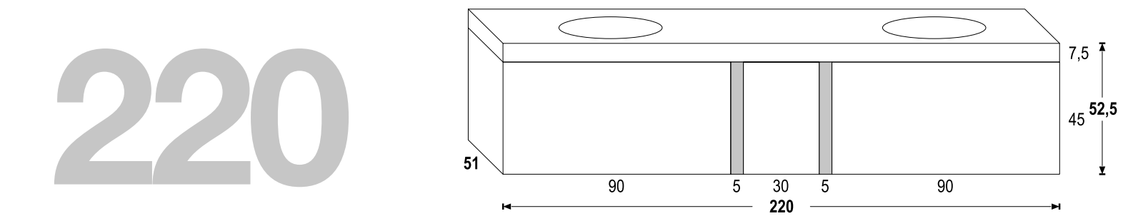
PORTALAVABO SOSPESO SENZA TOP - L. 220 P.51 H. 52,5 WALL-MOUNTED WASHBASIN CABINET WITHOUT TOP - W.220 D.51 H.52,5
