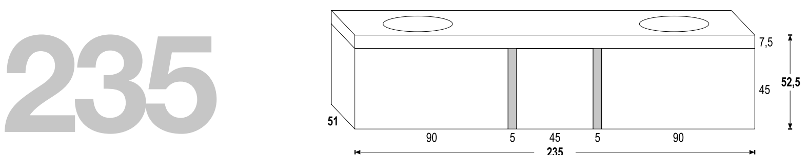
PORTALAVABO SOSPESO SENZA TOP - L. 235 P.51 H. 52,5 WALL-MOUNTED WASHBASIN CABINET WITHOUT TOP - W.235 D.51 H.52,5
