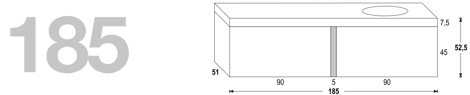
PORTALAVABO SOSPESO SENZA TOP - L. 185 P.51 H. 52,5 WALL-MOUNTED WASHBASIN CABINET WITHOUT TOP - W.185 D.51 H.52,5
