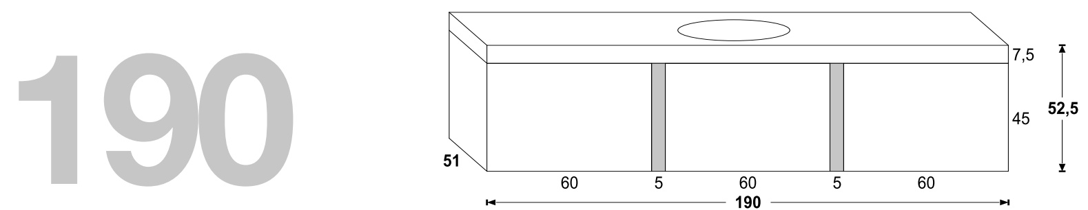
PORTALAVABO SOSPESO SENZA TOP - L. 190 P.51 H. 52,5 WALL-MOUNTED WASHBASIN CABINET WITHOUT TOP - W.190 D.51 H.52,5
