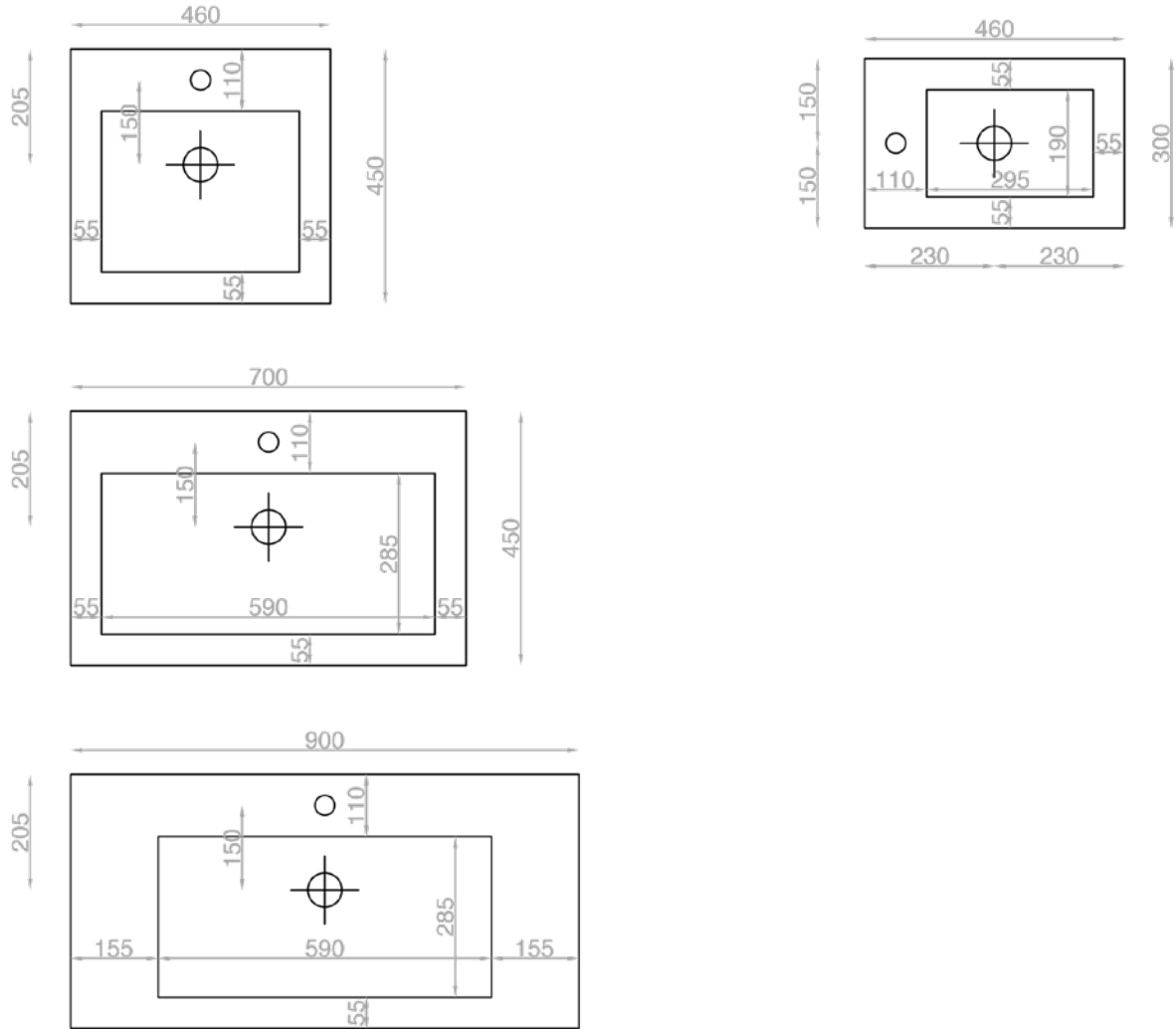
LAVABI MUTEVOLE - VISTA IN PIANTA MUTEVOLE BASINS - PLAN VIEW
