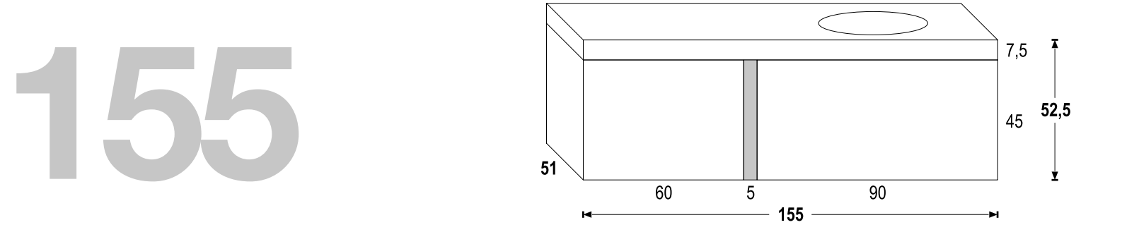
PORTALAVABO SOSPESO SENZA TOP - L. 155 P.51 H. 52,5 WALL-MOUNTED WASHBASIN CABINET WITHOUT TOP - W.155 D.51 H.52,5
