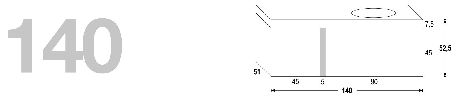
PORTALAVABO SOSPESO SENZA TOP - L. 140 P.51 H. 52,5 WALL-MOUNTED WASHBASIN CABINET WITHOUT TOP - W.140 D.51 H.52,5
