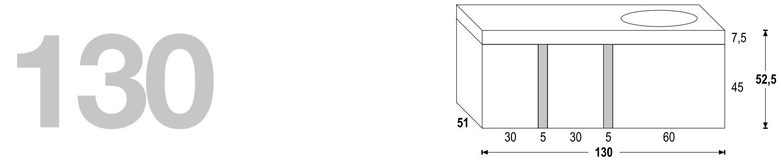
PORTALAVABO SOSPESO SENZA TOP - L. 130 P.51 H. 52,5 WALL-MOUNTED WASHBASIN CABINET WITHOUT TOP - W.130 D.51 H.52,5
