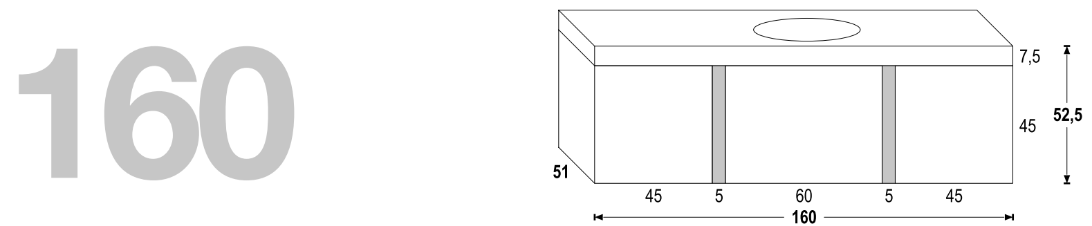
PORTALAVABO SOSPESO SENZA TOP - L. 160 P.51 H. 52,5 WALL-MOUNTED WASHBASIN CABINET WITHOUT TOP - W.160 D.51 H.52,5
