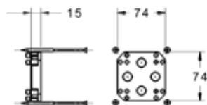
649.41.360 Адаптер-удлинитель
