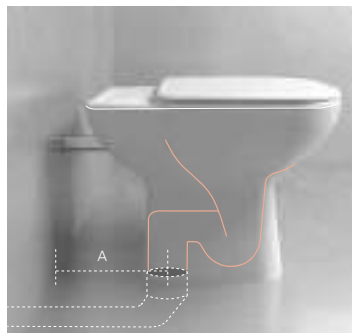
Vaso tradizionale scarico a terra Traditional floor outlet wc
