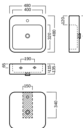
Apertura per installazione su piano Hole for surface installation
