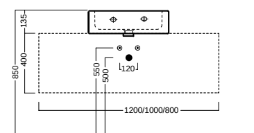
Apertura per installazione su piano Hole for surface installation
