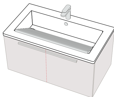
// Lavabo 04 1.91 x p.52 cm interno vasca: 75 x 36 x 17 cm
