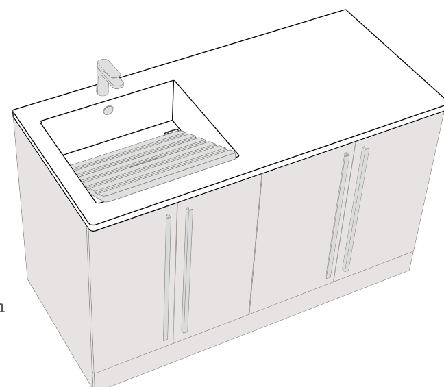
// Lavabo porta lavatrice SX 1.130 x p.62 cm interno vasca: 51 x 46 x 17 cm piano laterale: 75 x 62 cm
