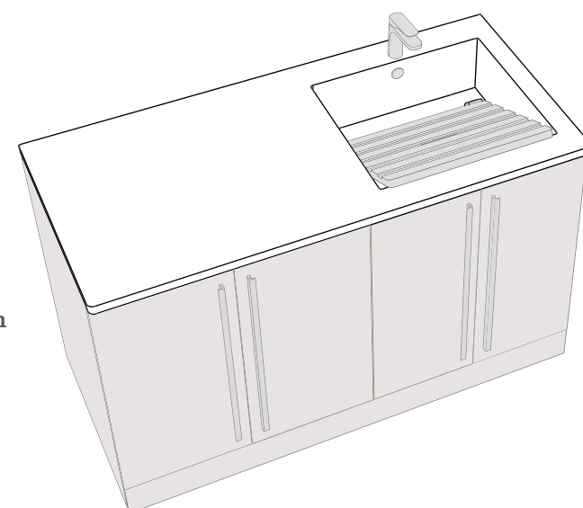
// Lavabo porta lavatrice DX 1.130 x p.62 cm interno vasca: 51 x 46 x 17 cm piano laterale: 75 x 62 cm
