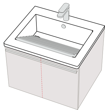
// Lavabo 01 1.61 x p.52 cm interno vasca: 51 x 36 x 17 cm
