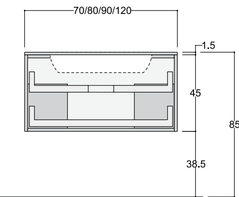
CONSOLLE O LAVABO SOTTOPIANO
