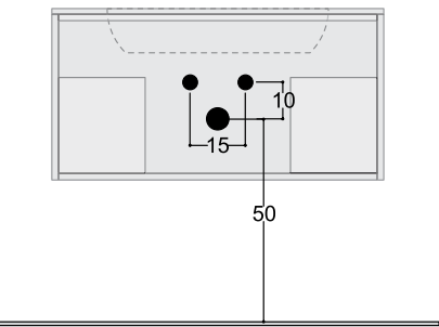
POSIZIONE SCARICHI
