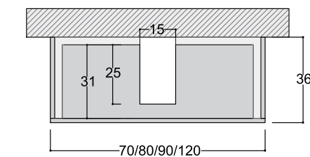
VISTA IN PIANTA CASSETTO ASOLATO P. 36
