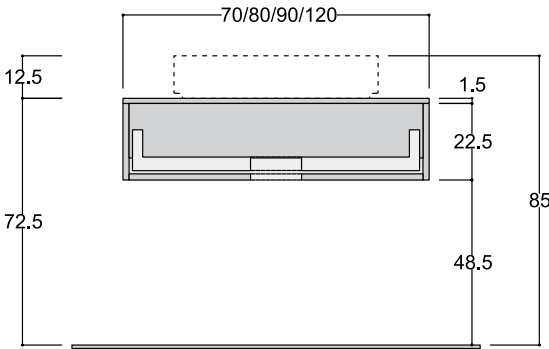
LAVABO DA APPOGGIO TUTTO FUORI
