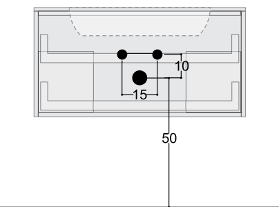
POSIZIONE SCARICHI
