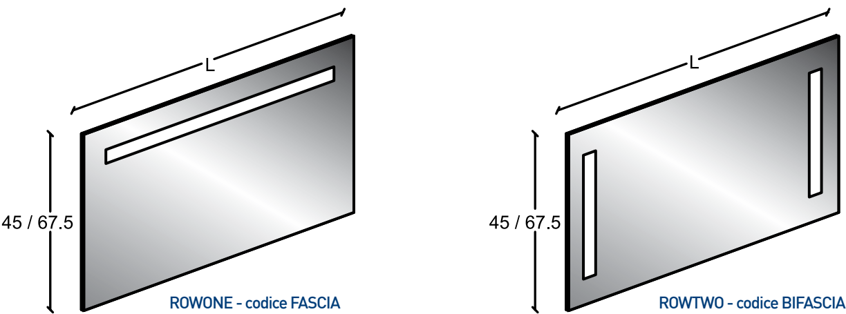
Specchiere Rowone e Rowtwo filo lucido - Fascia satinata retroilluminata led - Telaio PVC finitura cromo Sp. 2,5 cm - Dotate di interruttore sul telaio inferiore
