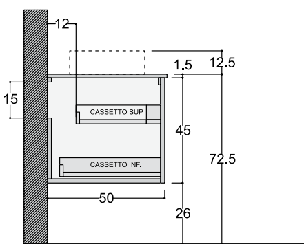
VISTA LATERALE P. 50
