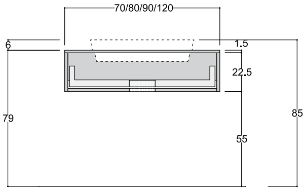
LAVABO SOPRAPIANO INCASSO PARZIALE
