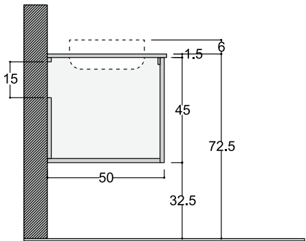
VISTA LATERALE P. 50
