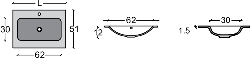
DIMENSIONI VASCA
