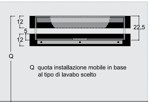
SCHEMA INSTALLAZIONE RINFORZI
