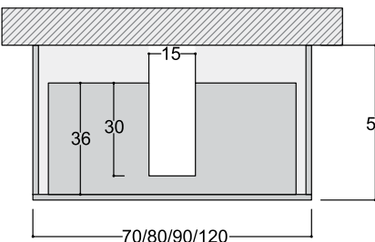
VISTA IN PIANTA CASSETTO ASOLATO P. 50
