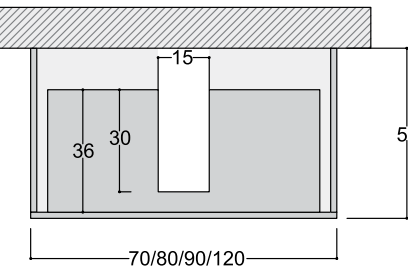
VISTA IN PIANTA CASSETTO ASOLATO P. 50
