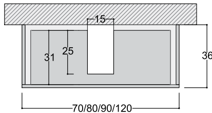
VISTA IN PIANTA CASSETTO ASOLATO P. 36
