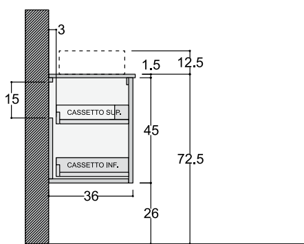
VISTA LATERALE P. 36
