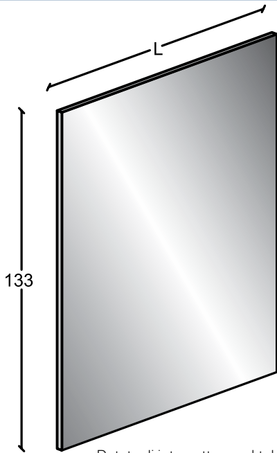
Specchiera All filo lucido - Telaio PVC finitura grigio Sp. 2,5 cm Dotata di interruttore sul telaio inferiore - Disponibile a misura in larghezza
