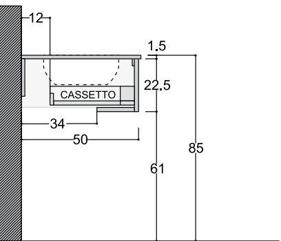
VISTA LATERALE P. 50
