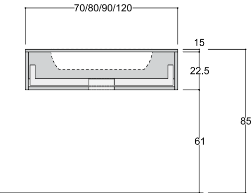
CONSOLLE O LAVABO SOTTOPIANO
