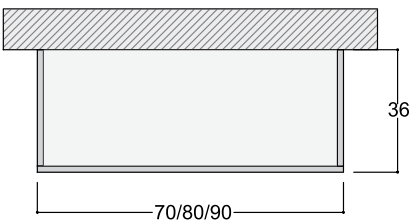
VISTA IN PIANTA P. 36
