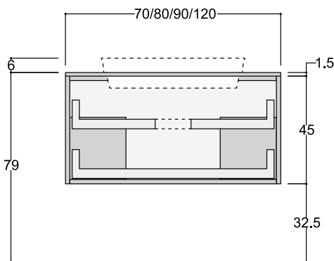
LAVABO SOPRAPIANO INCASSO PARZIALE
