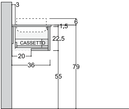
VISTA LATERALE P. 36
