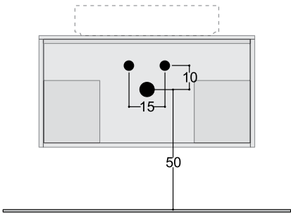
POSIZIONE SCARICHI
