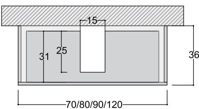
VISTA IN PIANTA CASSETTO ASOLATO P. 36
