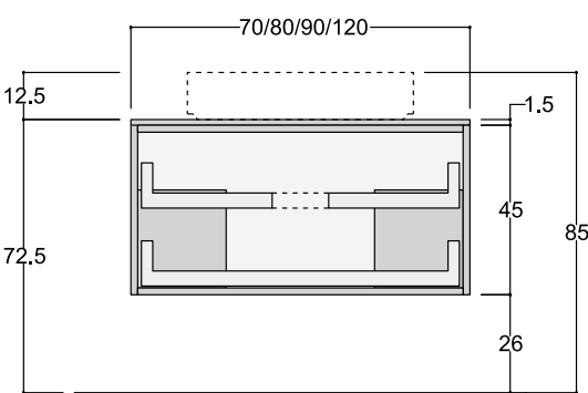
LAVABO DA APPOGGIO TUTTO FUORI
