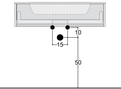
POSIZIONE SCARICHI
