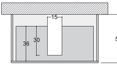
VISTA IN PIANTA CASSETTO ASOLATO P. 50
