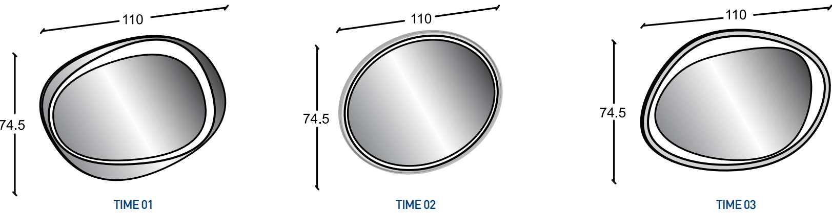
Specchiere Time 01, Time 02 e Time 03 filo lucido - Fascia satinata retroilluminata led - Telaio in legno Sp. 2 cm - Dotate di interruttore
