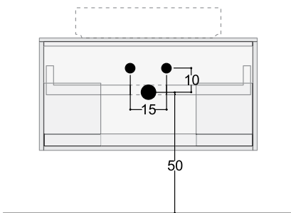
POSIZIONE SCARICHI
