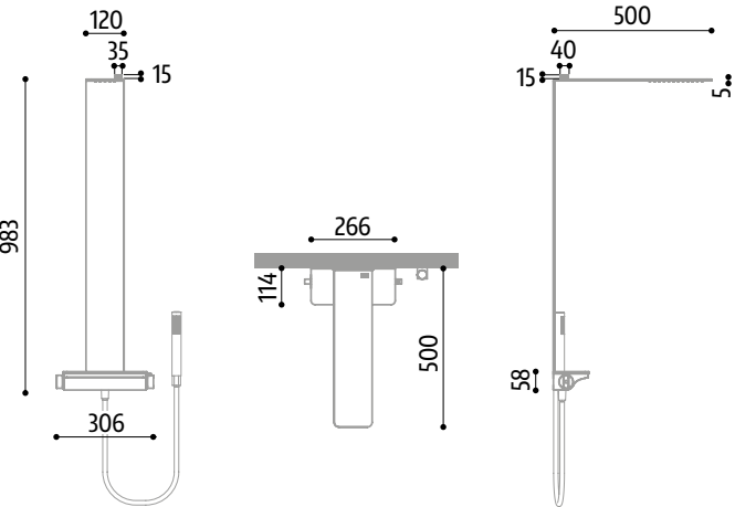
misure espresse in mm les dimensions sont en mm dimensions in mm
