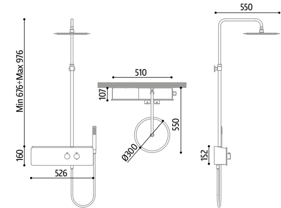
misure espresse in mm les dimensions sont en mm dimensions in mm
