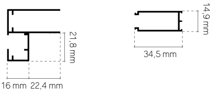
profilo compensatore e murale profilé de compensation et mural
