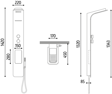
misure espresse in mm les dimensions sont en mm dimensions in mm
