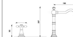
SBLV-DD-xx BATTERIA LAVABO TRE FORI THREE HOLES MIXER FOR WASHBASIN СМЕСИТЕЛЬ ДЛЯ РАКОВИНЫ НА 3 ОТВ.
