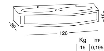
BSD-126 BASE P/LAVABO DOPPIA SOSPESA HANGING BASE FOR TWO WASHBASINS ТУМБА НАВЕСНАЯ ПОД ДВЕ РАКОВИНЫ
