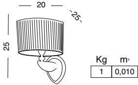
FH-FP01 FARETTO A PARETE CON PARALUME BIANCO O NERO WALL SPOTLIGHT WITH LAMP SHADE WHITE OR BLACK БРА НАСТЕННОЕ С АБАЖУРОМ БЕЛЫЙ - ЧЕРНЫЙ
