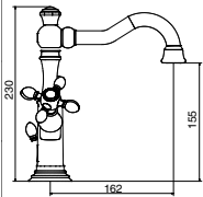
SMLV-BB-xx MONOFORO LAVABO SINGLE HOLE MIXER FOR WASHBASIN СМЕСИТЕЛЬ ДЛЯ РАКОВИНЫ НА 1 ОТВ.
