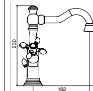
SMLV-TT-xx MONOFORO LAVABO SINGLE HOLE MIXER FOR WASHBASIN СМЕСИТЕЛЬ ДЛЯ РАКОВИНЫ НА 1 ОТВ.
