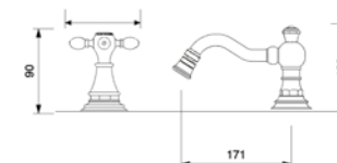
SBDT-AA-xx BATTERIA BIDET TRE FORI THREE HOLES MIXER FOR BIDET СМЕСИТЕЛЬ ДЛЯ БИДЕ НА 3 ОТВ.
