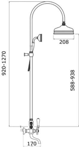
SGVD-DD-xx GRUPPO VASCA/DOCCIA ESTERNO CON SOFFIONE E DOCCETTA EXTERNAL SET FOR BATHTUB SHOWER WITH SHOWER HEAD AND HANDSHOWER СМЕСИТЕЛЬ ДЛЯ ВАННЫ/ДУША С ВНЕШНЕЙ ТРУБКОЙ, ИЗЛИВОМ, ВЕРХНИМ И РУЧНЫМ ДУШЕМ
