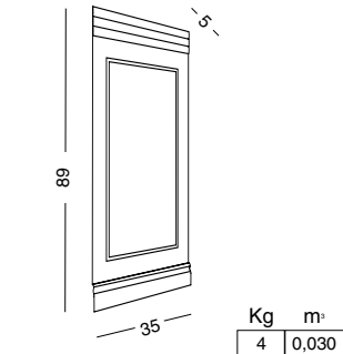
BPBB-35 BOISERIE 35 BASSA LOW BOISERIE 35 НБУАЗЕРИ 35 НИЖНЯЯ
