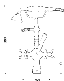
SGVE-DD-xx GRUPPO VASCA ESTERNO EXTERNAL SET FOR BATHTUB СМЕСИТЕЛЬ ДЛЯ ВАННЫ ВНЕШНИЙ С РУЧНЫМ ДУШЕМ
