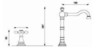
SBLV-BB-xx BATTERIA LAVABO TRE FORI THREE HOLES MIXER FOR WASHBASIN СМЕСИТЕЛЬ ДЛЯ РАКОВИНЫ НА 3 ОТВ.
