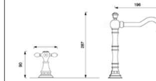
SBLV-TT-xx BATTERIA LAVABO TRE FORI THREE HOLES MIXER FOR WASHBASIN СМЕСИТЕЛЬ ДЛЯ РАКОВИНЫ НА 3 ОТВ.
