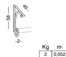
BST-25 STRUTTURA PORTANTE DX O SX PER P/LAVABI SOSPESI PREDISPOSTA PER ALLOGGIO MENSOLA VETRO SABBIAATO (BMN-84 E BMN-126) RIGHT-HAND OR LEFT-HAND SUPPORTING STRUCTURE FOR HANGING WASHBASIN BASE PRE-PUNCHED FOR SANDBLASTED GLASS SHELF (BMN-84 AND BMN-126) ПОДДЕРЖИВАЮЩИЙ ЭЛЕМЕНТ ДЛЯ НАВЕСНЫХ ТУМБ С ДЕРЖАТЕЛЕМ ДЛЯ ПОЛКИ ИЗ МАТОВОГО СТЕКЛА BMN-84 ИЛИ BMN-126 - DX/SX
