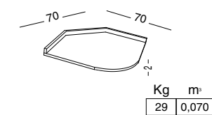
HGMA-700 PIANO BASE ANGOLARE DX O SX CON ALZATINA TOP WITH BACKSPLASH FOR ANGULAR WASHBASIN BASE (RIGHT-LEFT) ДЛЯ УГЛОВОЙ ТУМБЫ DX/SX С ПРИСТЕННОЙ ПЛАНКОЙ
