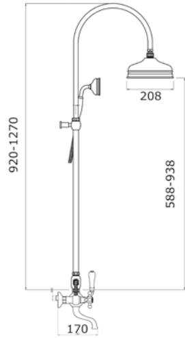
SGVD-BB-xx GRUPPO VASCA/DOCCIA ESTERNO CON SOFFIONE E DOCCETTA EXTERNAL SET FOR BATHTUB SHOWER WITH SHOWER HEAD AND HANDSHOWER СМЕСИТЕЛЬ ДЛЯ ВАННЫ/ДУША С ВНЕШНЕЙ ТРУБКОЙ, ИЗЛИВОМ, ВЕРХНИМ И РУЧНЫМ ДУШЕМ
