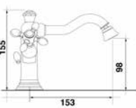
SMBD-BB-xx MONOFORO BIDET SINGLE HOLE MIXER FOR BIDE СМЕСИТЕЛЬ ДЛЯ БИДЕ НА 1 ОТВ.
