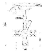
SGVE-BB-xx GRUPPO VASCA ESTERNO EXTERNAL SET FOR BATHTUB СМЕСИТЕЛЬ ДЛЯ ВАННЫ ВНЕШНИЙ С РУЧНЫМ ДУШЕМ
