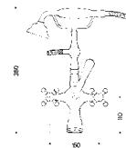
SGVE-AA-xx GRUPPO VASCA ESTERNO EXTERNAL SET FOR BATHTUB СМЕСИТЕЛЬ ДЛЯ ВАННЫ ВНЕШНИЙ С РУЧНЫМ ДУШЕМ
