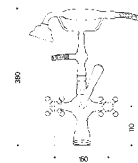
SGVE-TT-xx GRUPPO VASCA ESTERNO EXTERNAL SET FOR BATHTUB СМЕСИТЕЛЬ ДЛЯ ВАННЫ ВНЕШНИЙ С РУЧНЫМ ДУШЕМ
