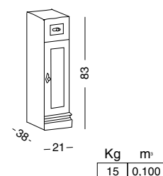
BAC-21 BASE RETTA 21 CON 1 CASSETTO E ANTA DX O SX BASE 21 WITH 1 DRAWER AND DOOR (RIGHT - LEFT) ТУМБА ПРЯМАЯ 21 С 1 ЯЩИКОМ И СТВОРКОЙ DX/SX
