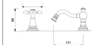
SBDT-DD-xx BATTERIA BIDET TRE FORI THREE HOLES MIXER FOR BIDET СМЕСИТЕЛЬ ДЛЯ БИДЕ НА 3 ОТВ.
