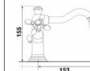
SMBD-CC-xx MONOFORO BIDET SINGLE HOLE MIXER FOR BIDE СМЕСИТЕЛЬ ДЛЯ БИДЕ НА 1 ОТВ.
