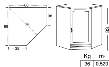
BAM-68 BASE ANGOLARE ANGULAR BASE ТУМБА УГЛОВАЯ
