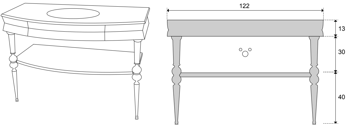
FASHION FH-M124G BASE P/LAVABO SINGOLO CON RIPIANO SOTTOSTANTE IN LEGNO E GAMBE METALLICHE BASE FOR ONE WASHBASIN WITH WOODEN SHELF AND METAL LEGS ТУМБА ПОД ОДНУ РАКОВИНУ С ДЕРЕВЯННОЙ ПОЛКОЙ И МЕТАЛЛИЧЕСКИМИ НОЖКАМИ
