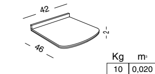
HGMC-42 PIANO CONSOLLE TRUCCO CON ALZATINA TOP WITH BACKSPLASH FOR MAKE-UP CONSOLE ДЛЯ КОСМЕТИЧЕСКОЙ КОНСОЛИ С ПРИСТЕННОЙ ПЛАНКОЙ
