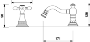
SBDT-BB-xx BATTERIA BIDET TRE FORI THREE HOLES MIXER FOR BIDET СМЕСИТЕЛЬ ДЛЯ БИДЕ НА 3 ОТВ.
