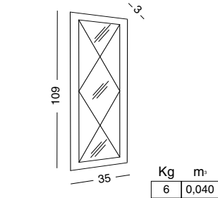
BPBA-35 BOISERIE 35 ALTA CON SPECCHIO A LOSANGHE HIGHT BOISERIE 35 AND MIRROR WITH LO-ZENGE DECOR БУАЗЕРИ 35 ВЕРХНЯЯ И ЗЕРКАЛО С РОМБОВИДНЫМ ДЕКОРОМ
