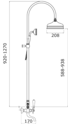
SGVD-TT-xx GRUPPO VASCA/DOCCIA ESTERNO CON SOFFIONE E DOCCETTA EXTERNAL SET FOR BATHTUB SHOWER WITH SHOWER HEAD AND HANDSHOWER СМЕСИТЕЛЬ ДЛЯ ВАННЫ/ДУША С ВНЕШНЕЙ ТРУБКОЙ, ИЗЛИВОМ, ВЕРХНИМ И РУЧНЫМ ДУШЕМ
