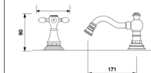
SBDT-CC-xx BATTERIA BIDET TRE FORI THREE HOLES MIXER FOR BIDET СМЕСИТЕЛЬ ДЛЯ БИДЕ НА 3 ОТВ.
