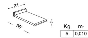
HGMR-21 PIANO BASE RETTA 21 CON ALZATINA TOP WITH BACKSPLASH FOR BASE 21 ДЛЯ ТУМБЫ ПРЯМОЙ 21 С ПРИСТЕННОЙ ПЛАНКОЙ
