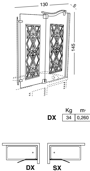
BOX-VAS PARETE SOPRA VASCA DX O SX WALL BATH SCREEN (RIGHT-LEFT) ДУШЕВАЯ ШТОРКА (УКАЗАТЬ ПРАВО/ЛЕВОСТОРОННЯЯ)
