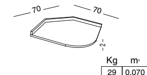
HGMA-700 PIANO BASE ANGOLARE DX O SX CON ALZATINA TOP WITH BACKSPLASH FOR ANGULAR WASHBASIN BASE (RIGHT-LEFT) ДЛЯ УГЛОВОЙ ТУМБЫ DX/SX С ПРИСТЕННОЙ ПЛАНКОЙ
