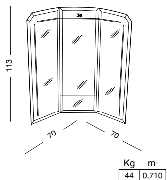
HGSA-70 SPECCHIERA CONTENITORE SENZA ILLUMINAZIONE CABINET MIRROR WITHOUT LIGHTING ЗЕРКАЛО УГЛОВОЕ СО ШКАФЧИКОМ, БЕЗ ПОДСВЕТКИ
