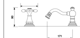
SBDT-CC-xx BATTERIA BIDET TRE FORI THREE HOLES MIXER FOR BIDET СМЕСИТЕЛЬ ДЛЯ БИДЕ НА 3 ОТВ.
