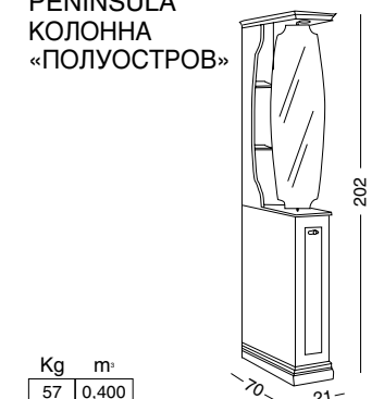
BPC-21 PENISOLA COMPLETA CON SPECCHIO GIREVOLE ATTREZZATO E FARETTO ALOGENO COMPLETE PENINSULA WITH ROTATING EQUIPPED MIRROR AND HALOGEN SPOTLIGHT КОЛОННА «ПОЛУОСТРОВ» С ПОВОРОТНЫМ ЗЕРКАЛОМ И ГАЛОГЕННЫМ СВЕТИЛЬНИКОМ
