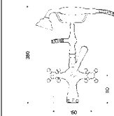
SGVE-BB-xx GRUPPO VASCA ESTERNO EXTERNAL SET FOR BATHTUB СМЕСИТЕЛЬ ДЛЯ ВАННЫ ВНЕШНИЙ С РУЧНЫМ ДУШЕМ
