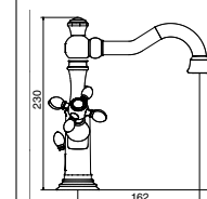
SMLV-CC-xx MONOFORO LAVABO SINGLE HOLE MIXER FOR WASHBASIN СМЕСИТЕЛЬ ДЛЯ РАКОВИНЫ НА 1 ОТВ.
