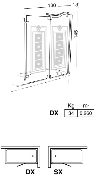
C-BOX-VAS PARETE SOPRA VASCA DX O SX WALL BATH SCREEN (RIGHT-LEFT) ДУШЕВОЕ ОГРАЖДЕНИЕ ДЛЯ УСТАНОВКИ НА ВАННУ DX/SX
