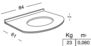
HGMS-84 PIANO P/LAV. SINGOLO CON ALZATINA TOP WITH BACKSPLASH FOR ONE WASHBASIN BASE ДЛЯ ТУМБЫ ПОД ОДНУ РАКОВИНУ С ПРИСТЕННОЙ ПЛАНКОЙ
