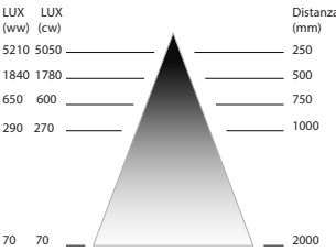
Diagramma di distribuzione luce
