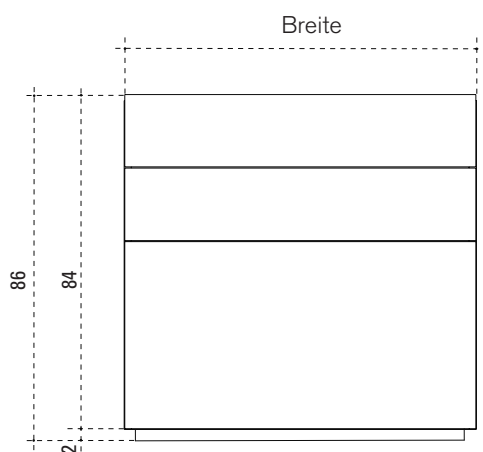
VORDERANSICHT
