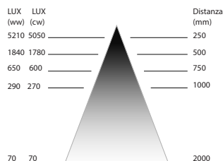
Diagramma di distribuzione luce
