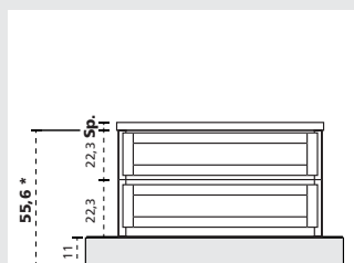
Panchetta a terra con basi in appoggio.
