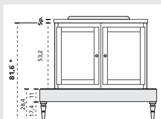
Base lavabo con lavabo integrale (o piano con vasca integrata o con lavabo sottopiano) e panchetta con piedini H.17,4 cm.
