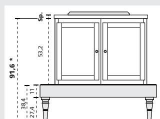
Base lavabo con lavabo integrale (o piano con vasca integrata o lavabo sottopiano) e panchetta con piedini H.27,4 cm.
