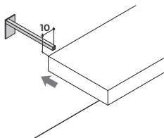
STAFFA PER MENSOLONE BRACKET FOR TOP IN HIGH THICKNESS КРОНШТЕЙН ДЛЯ БОЛЬШОЙ ПОЛКИ
