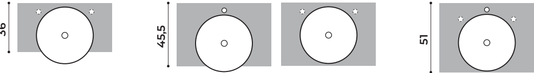
ALA P60 07 lavabo FONTE 60 / FONTE 60 basin / раковина FONTE 60
