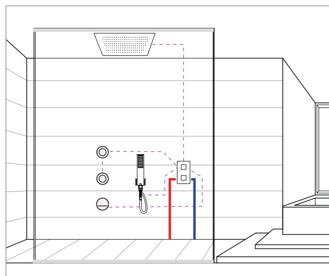
4 4 USCITE WAYS 4 OUTLETS
