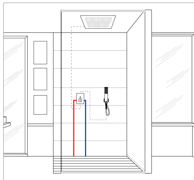
2 2 USCITE WAYS 2 OUTLETS
