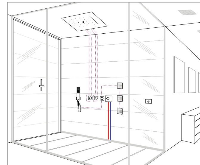
6 WAYS 6 USCITE: 3 deviatori con 6 vie 6 OUTLETS: Nr. 3 2-ways diverters
