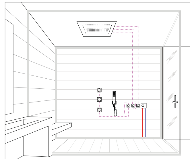
5 WAYS 5 USCITE: 2 deviatori con 2 vie + 1 via singola 5 OUTLETS: Nr. 2 2-ways diverters + 1 single way
