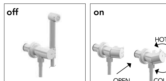
GANCIO DOCCETTA BIDET COMPLETO CON MISCELATORE INTEGRATO COMPLETE HOOK HAND SHOWER BIDET WITH INTEGRATE MIXER ART. 0403/MI/E, 7503/MI/E, 0303/MI/E, 1403/MI/E
