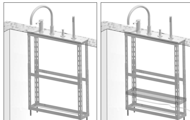
C - BORDO V-BOX CON PIASTRA A VISTA IN FINITURA. OPTIONAL: SISTEMA DI PRE-INSTALLAZIONE (012/6) E VASCHETTA DI RACCOLTA (012/7) C - BORDO V-BOX WITH AT SIGHT FINISHED PLATE. OPTIONAL: PRE-INSTALLATION SYSTEM (012/6) AND COLLECTION CASE (012/7)
