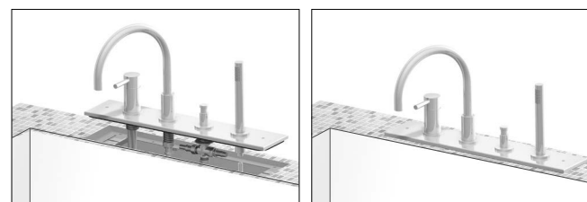
B - BORDO V-BOX CON PIASTRA A VISTA IN FINITURA. OPTIONAL: SISTEMA DI PRE-INSTALLAZIONE (012/6) B - BORDO V-BOX WITH AT SIGHT FINISHED PLATE. OPTIONAL: PRE-INSTALLATION SYSTEM (012/6)
