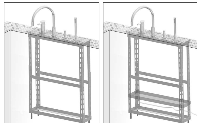
C - BORDO V-BOX CON PIASTRA RIVESTITA. OPTIONAL: SISTEMA DI PRE-INSTALLAZIONE (012/6) E VASCHETTA DI RACCOLTA (012/7) C - BORDO V-BOX WITH FACED PLATE. OPTIONAL: PRE-INSTALLATION SYSTEM (012/6) AND COLLECTION CASE (012/7)
