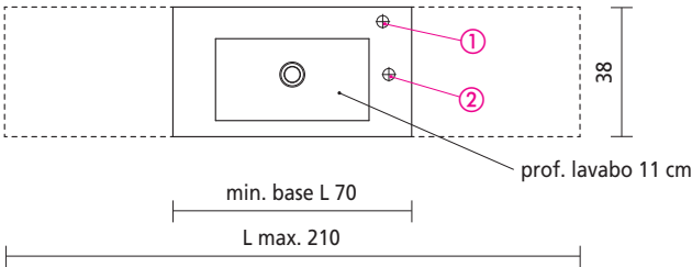
VASCA SINGOLA LAVABO TIME Misure interne: L 46 x P 23 x H 11 cm
