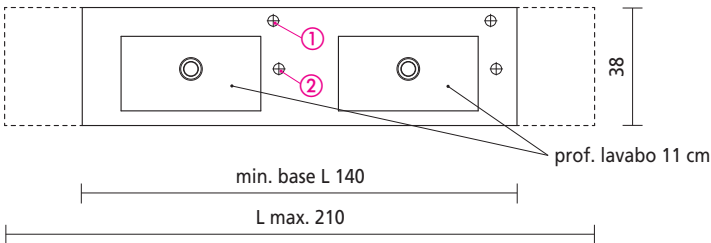
VASCA DOPPIA LAVABO TIME Misure interne: L 46 x P 23 x H 11 cm
