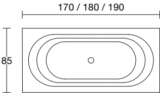
art. OASI33M - art. OASI34MC - art. OASI35MC
