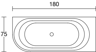
art. OASI51S VERSIONE SX-Left version-Version links- Version gauche-Versión izquierda-Левосторонний вариант
