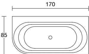
art. OASI53S VERSIONE SX-Left version-Version links- Version gauche-Versión izquierda-Левосторонний вариант
