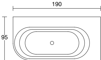
art. OASI58S VERSIONE SX-Left version-Version links- Version gauche-Versión izquierda-Левосторонний вариант
