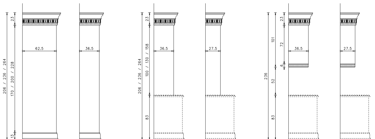
Grafico larghezze delle colonne, alzate, pensili / Graphic of the widths
