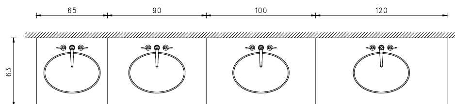
Grafico larghezze basi lavello / Graphic of the widths
