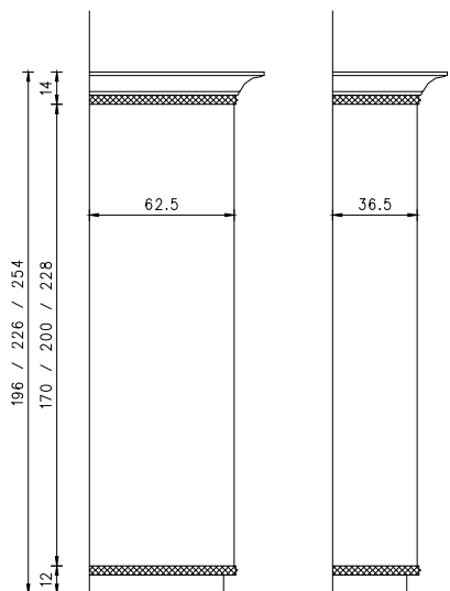
Grafico larghezze delle colonne, alzate, pensili / Graphic of the widths
