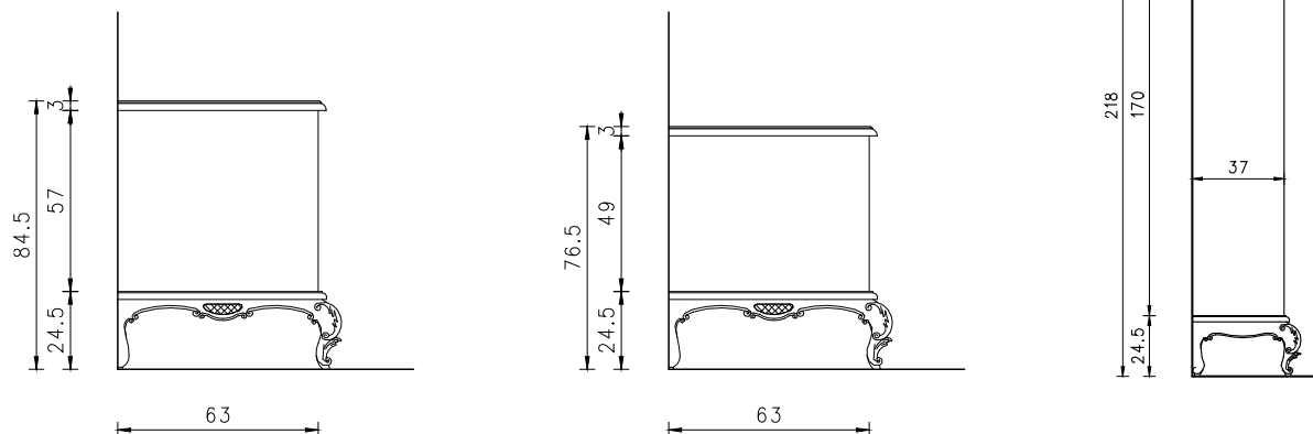
Grafico larghezze delle basi e colonne / Graphic of the widths
