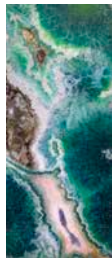
Reef
