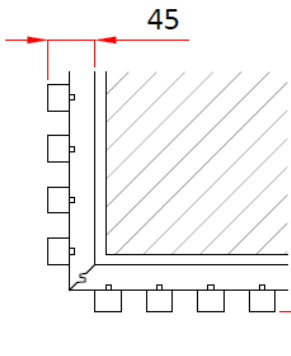
ANGOLO ESPOSTO 90° T25 – T25
