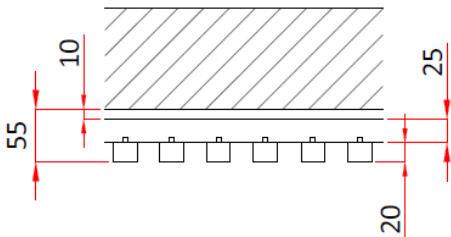
INFINITY T25 PANNELLO COMPLANARE ALLE PORTE
