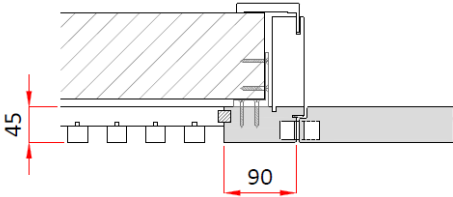
ELEMENTO MINIMO PER GIUNZIONE T25 – PORTA INFINTY 45 COMPLANARI
