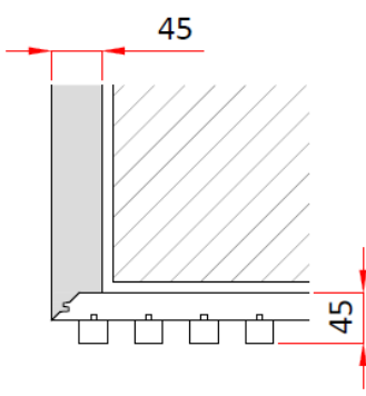
ANGOLO ESPOSTO 90° T25 – INFINITY 45
