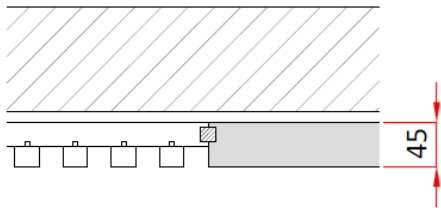
GIUNZIONE LINEARE T25 – INFINITY 45
