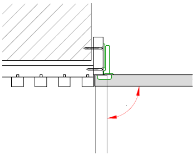
GIUNZIONE T25 – ANTA GUARDAROBA 25
