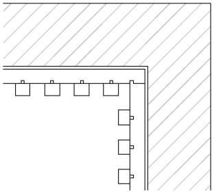
ANGOLO INTERNO 90° T25 – T25
