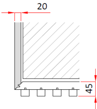
ANGOLO ESPOSTO 90° T25 – INFINITY 20
