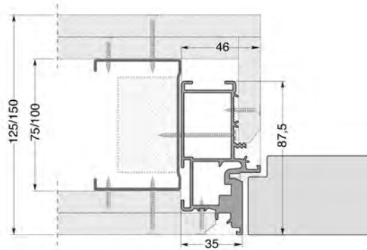
Parete cartongesso 125/150mm orditura 75/100 lastra doppia
