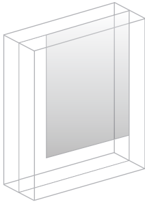
VETRO SABBIAITO 4/4 ACCOSTATO composto da 2 lastre temperate 4mm di cui una sabbiaita con perimetro trasparente
