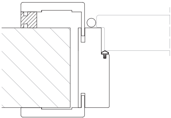
APPLICAZIONE DIETRO IL COPRIFILO
