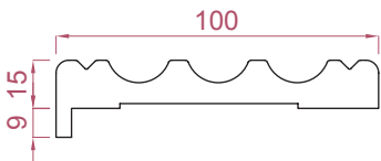
COPRIFILO ROMANICO 100x15 aletta 9mm Stipite BORDOPIANO Legno massello
