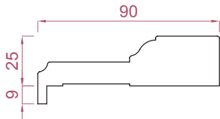
COPRIFILO TUSCANY 90x25 aletta 9mm Stipite BORDOPIANO Legno massello
