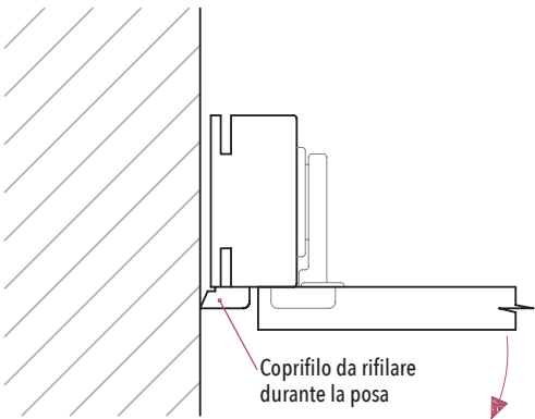
TELESCOPICO PARETE PERPENDICOLARE
