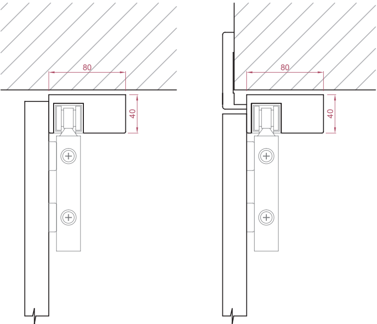
DETTAGLIO TRAVERSO BI-FOLD PER TUTTI I TIPI DI STIPITE
