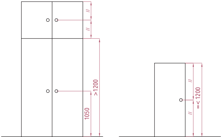
POSIZIONE STANDARD MANIGLIETTE AD INCASSO
