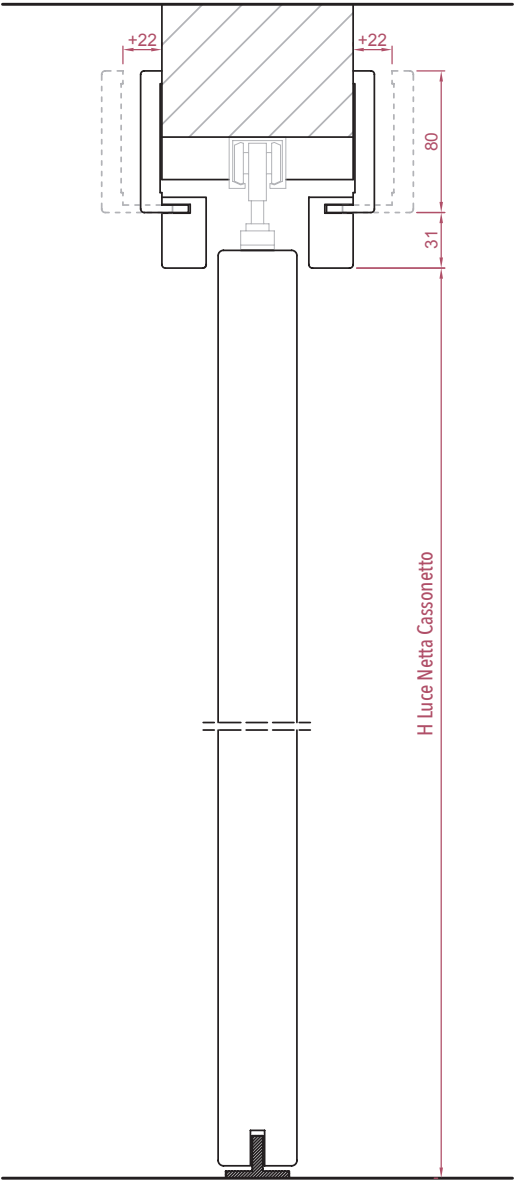
TIPO STIPITE BORDOPIANO
