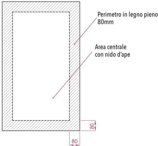
STRUTTURA ANTA TAMBURATA 25mm
