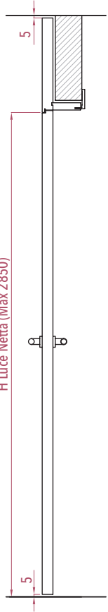
PORTA AD ALTEZZA RIDOTTA
