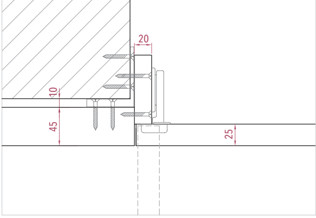
NODO INFINITY 45 - GUARDAROBA 25
