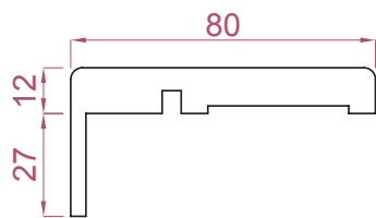
COPRIFILO 80x12 aletta 27mm Stipiti: BORDOPIANO / PIVOT / HF / REVERSE Legno multistrato impiallacciato
