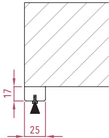
FASCETTA CON SPAZZOLINO A PARETE 25x17mm
