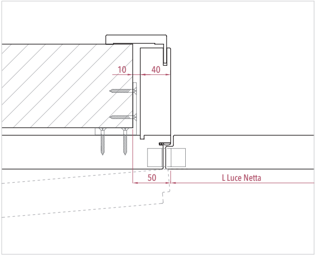
INFINITY - PORTA A TIRARE
