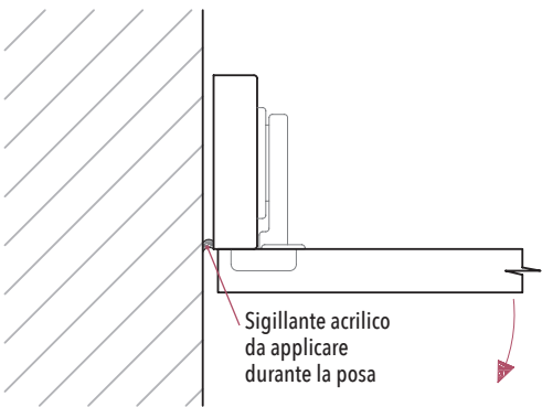
SLIM PARETE PERPENDICOLARE
