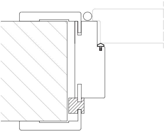
APPLICAZIONE A SPINGERE
