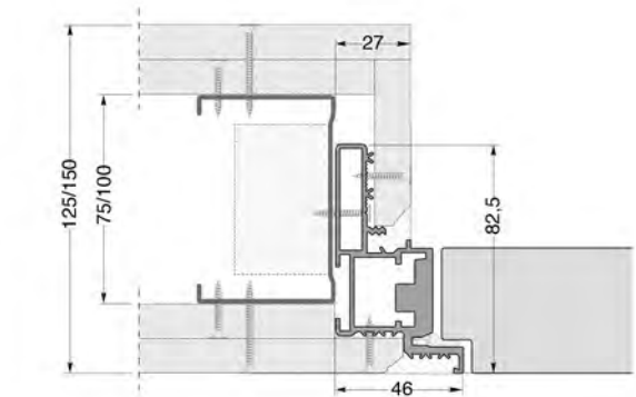
Parete cartongesso 125/150mm orditura 75/100 lastra doppia
