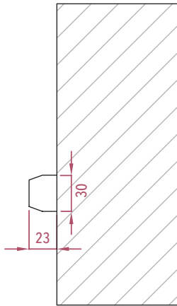
FASCETTA BATTUTA A PARETE 23x30mm
