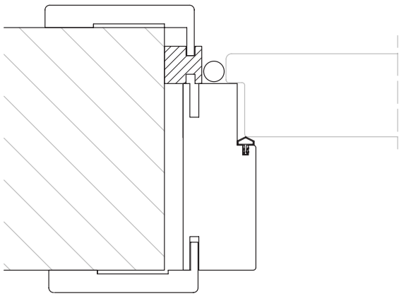
APPLICAZIONE A TIRARE
