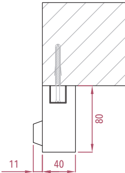
MONTANTE BATTUTA A PARETE 40x80mm
