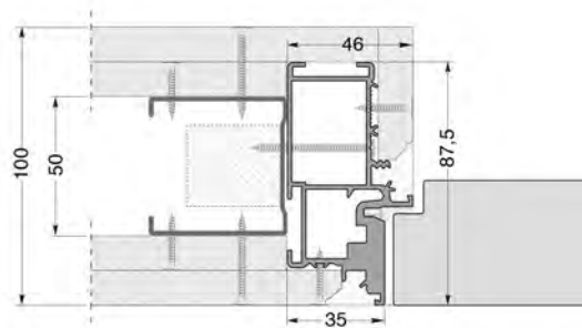
Parete cartongesso 100mm orditura 50 lastra doppia
