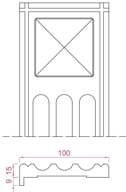
COPRIFILO ELLENICO 100x15 aletta 9mm CON PUNTA DI DIAMANTE Stipite BORDOPIANO Legno massello
