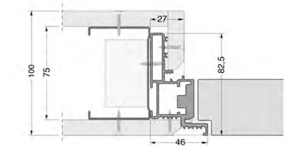
Parete cartongesso 100mm orditura 75 lastra singola
