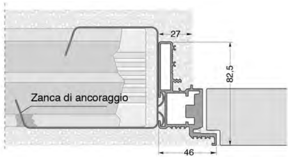
Parete intonacata spessore muro minimo 100mm
