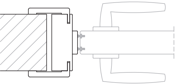
STIPITE PIVOT / HF / REVERSE
