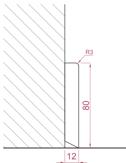
BATTISCOPIA LISCIO 80x12 Legno multistrato impiallacciato Lunghezza barre 2400mm
