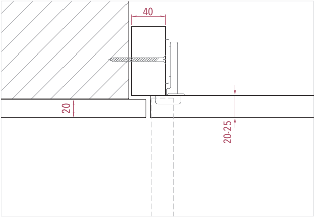
NODO INFINITY 20 - GUARDAROBA 20 / 25
