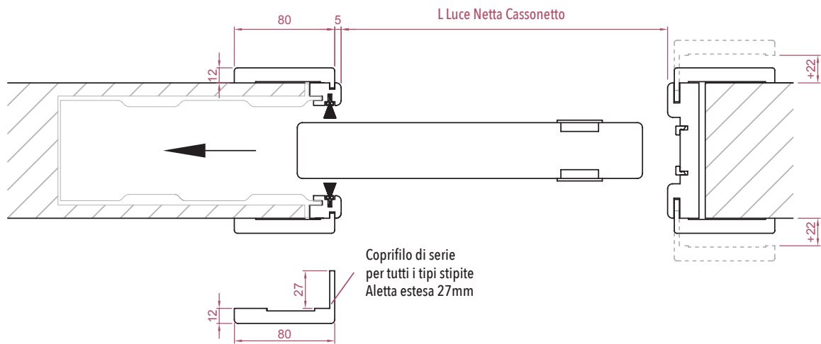
TIPI STIPITE BORDOPIANO / PIVOT / HF / REVERSE
