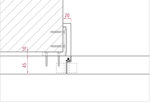
NODO BATTENTE INFINITY SENZA STIPITE
