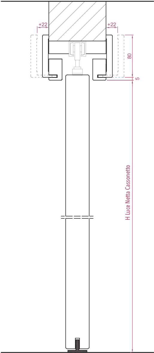
TIPI STIPITE PIVOT / HF / REVERSE
