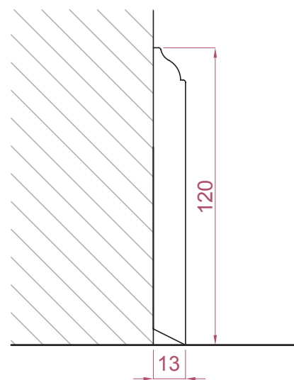
BATTISCOPIA TUSCANY 120x13 Legno massello Lunghezza barre variabile 1800-2700mm
