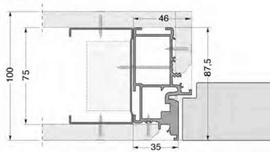
Parete cartongesso 100mm orditura 75 lastra singola
