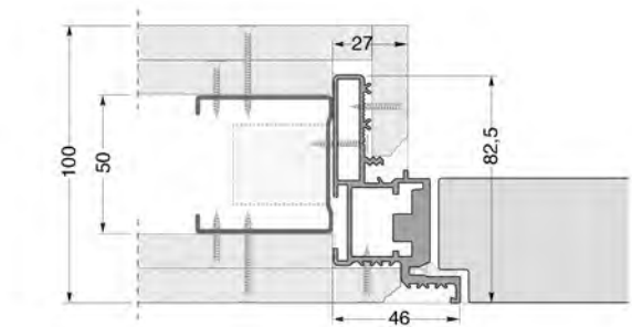
Parete cartongesso 100mm orditura 50 lastra doppia
