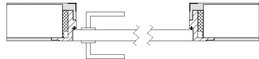
1-flügelig
