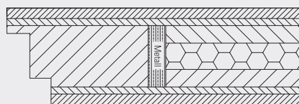
Beispiel: Tür GT.01, gefälzt mit Laibungsfalz, für Einfachzarge
