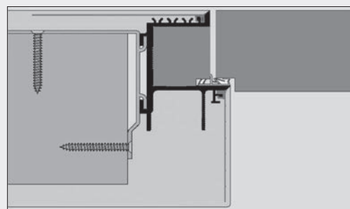
stumpf einschlagend (AGS TUT 45)
