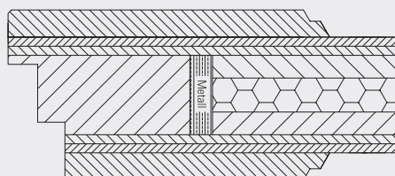
Beispiel: Tür Stilisten, gefälzt mit Laibungsfalz, für Einfachzarge
