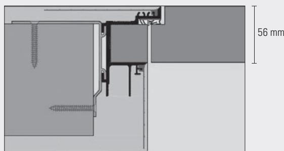
stumpf einschlagend, revers in die Laibung öffnend (AGS TUS 56)
