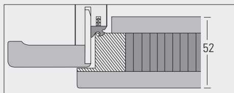
Tür gefälzt mit Laibungsfalz
