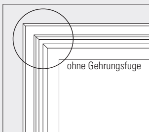
Beispiel: Zarge LD
