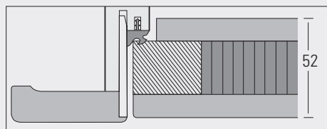
Tür stumpf mit Laibungsfalz
